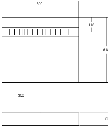
KL BASIN 600 W x 510 D x 100 H
